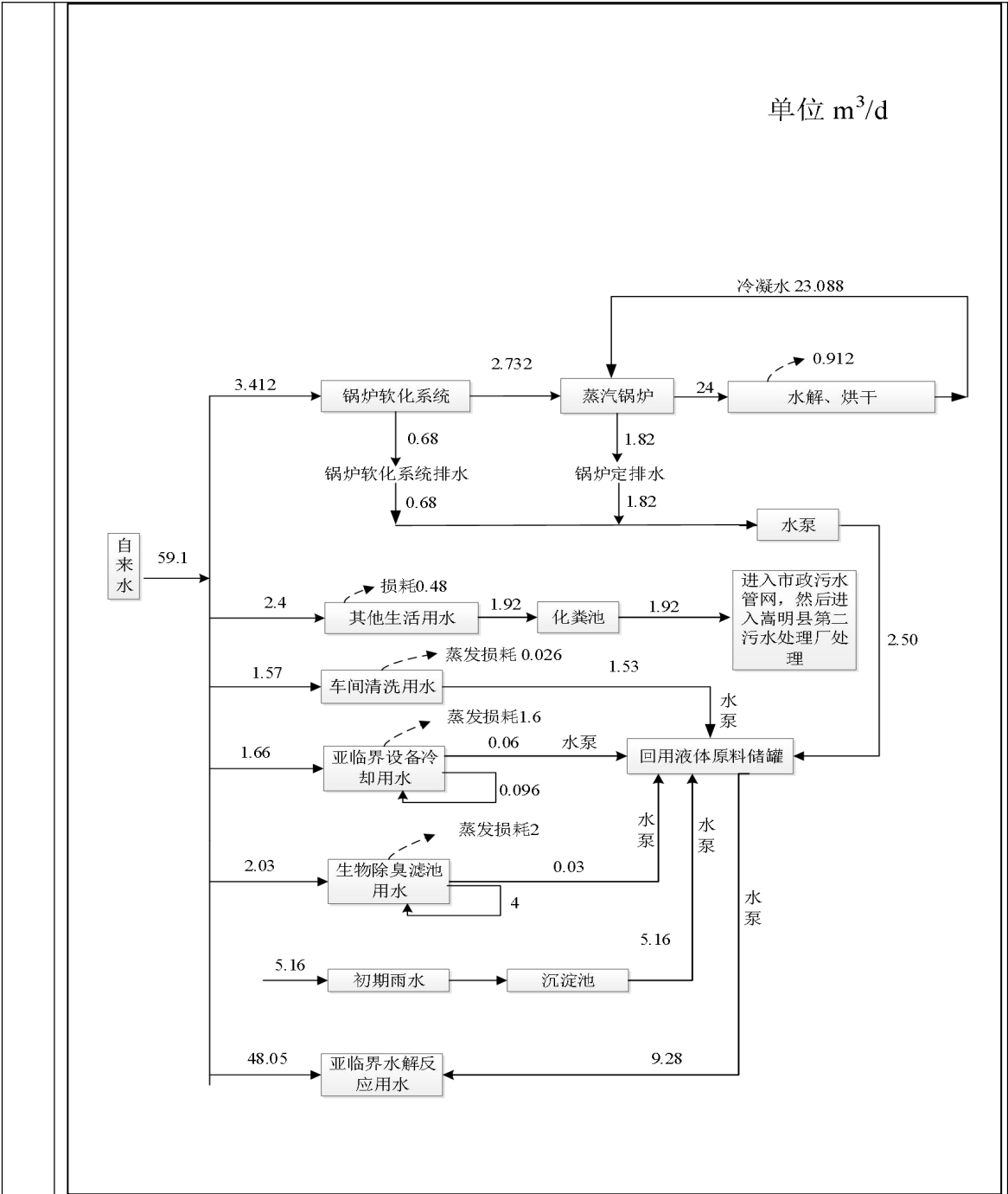
图 2-2 项目水量平衡图
