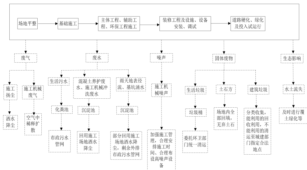
图 2-2 项目施工期工艺流程及产污节点示意图
