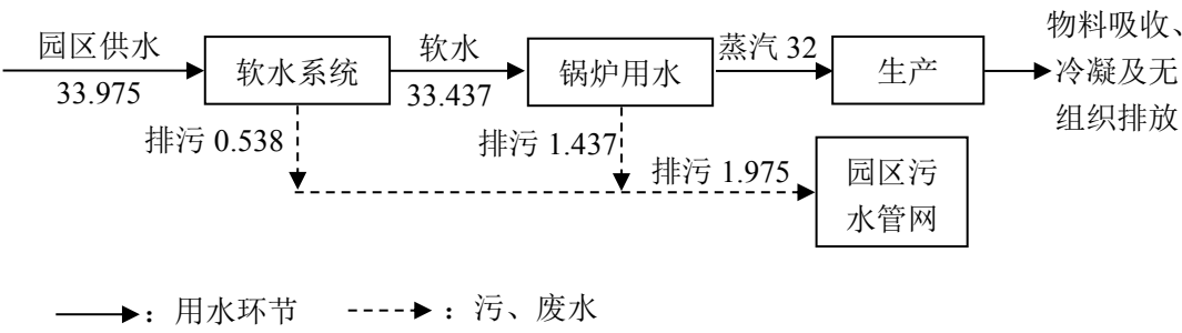
图 2-1 本项目水量平衡图 单位：m³/d
