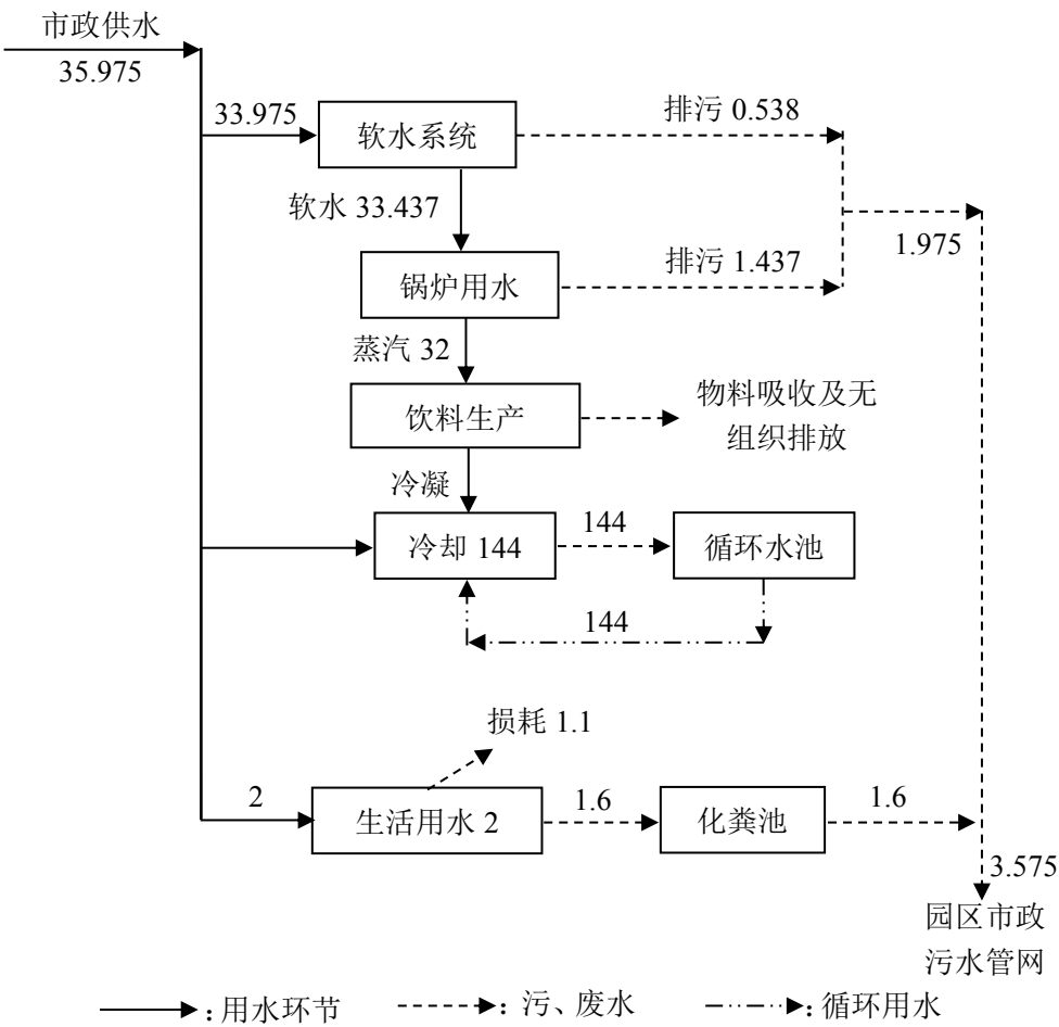
图 2-2 项目实施后全厂水量平衡图 单位：m³/d
