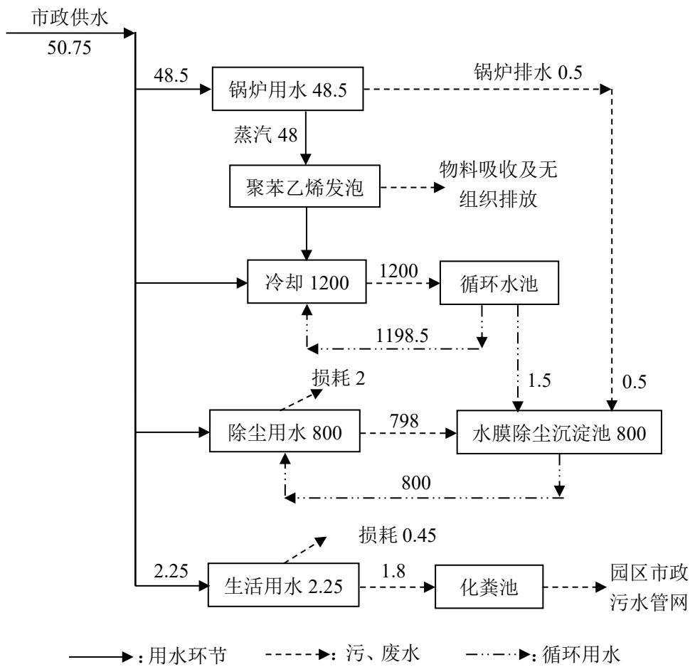
图 2-5 原有项目水量平衡图
