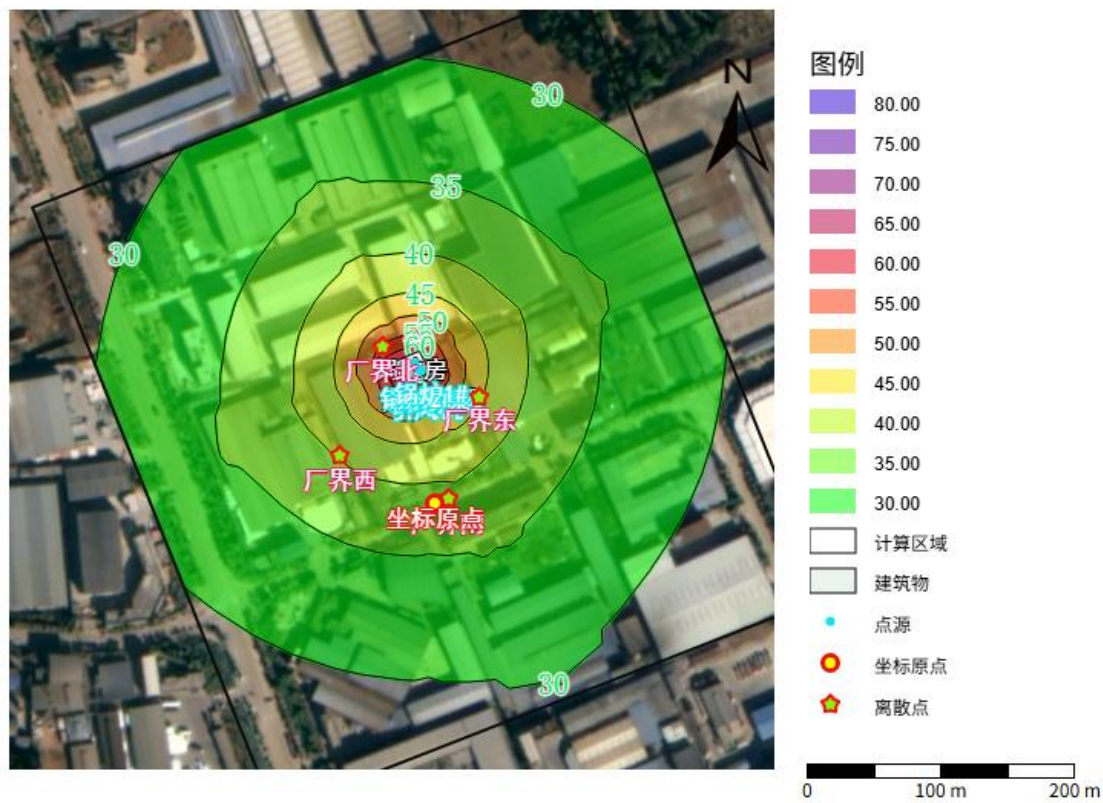
图 4-2 本项目厂界噪声（昼间）等值线图
