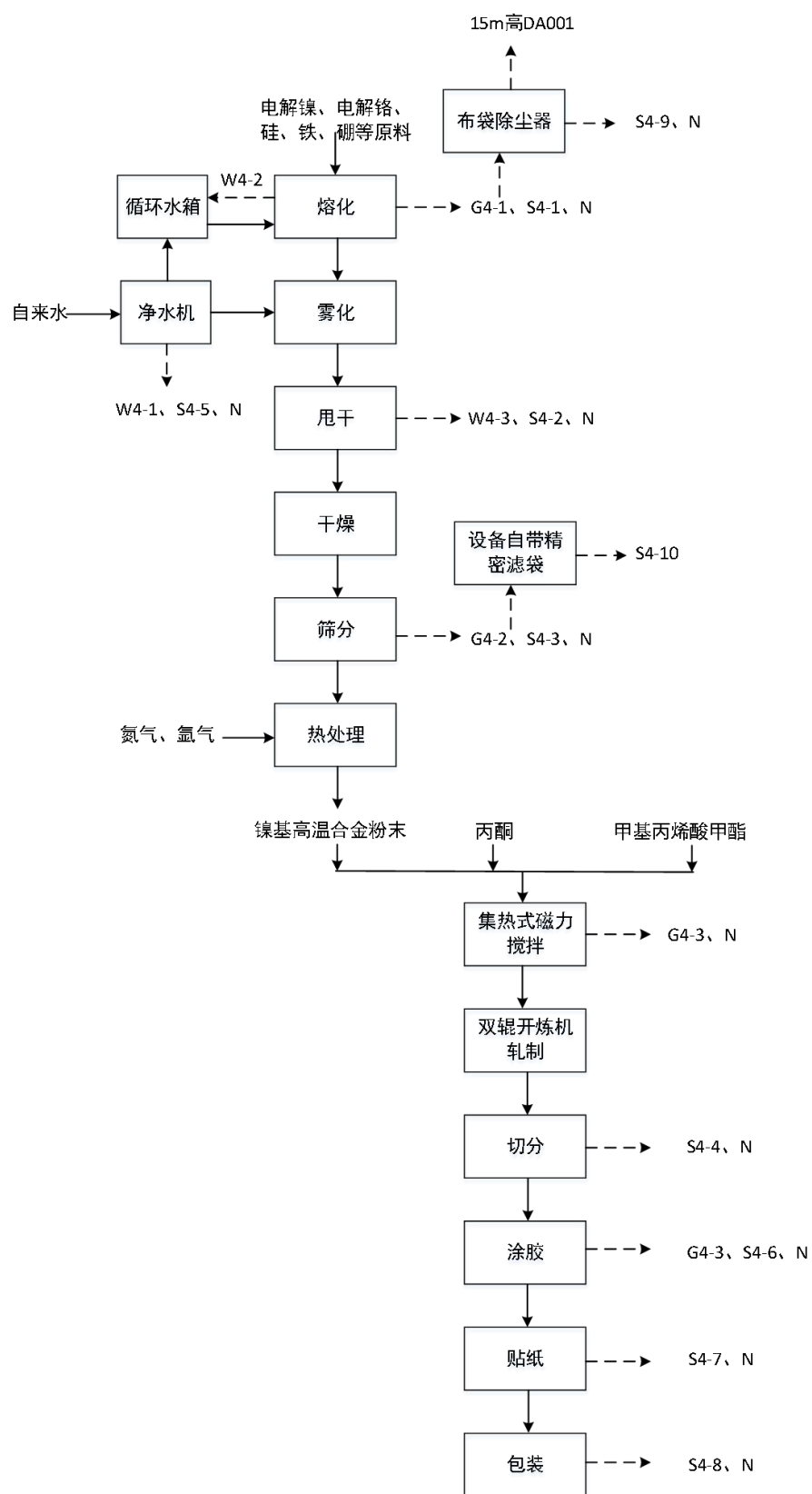
图 2-4 粘带生产工艺流程图
