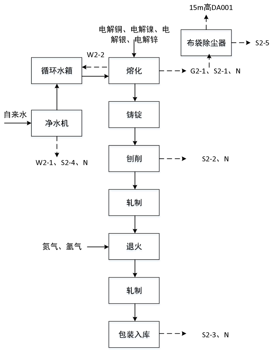
图 2-4 合金焊料片材生产工艺流程图
