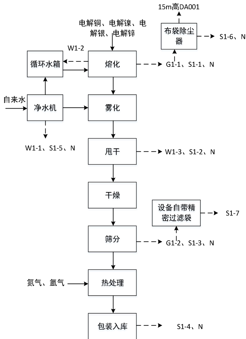
图 2-3 铜合金粉末生产工艺流程图
