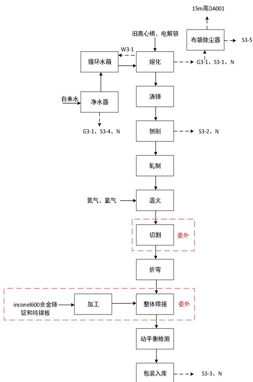
图 2-4 离心桶生产工艺流程图
