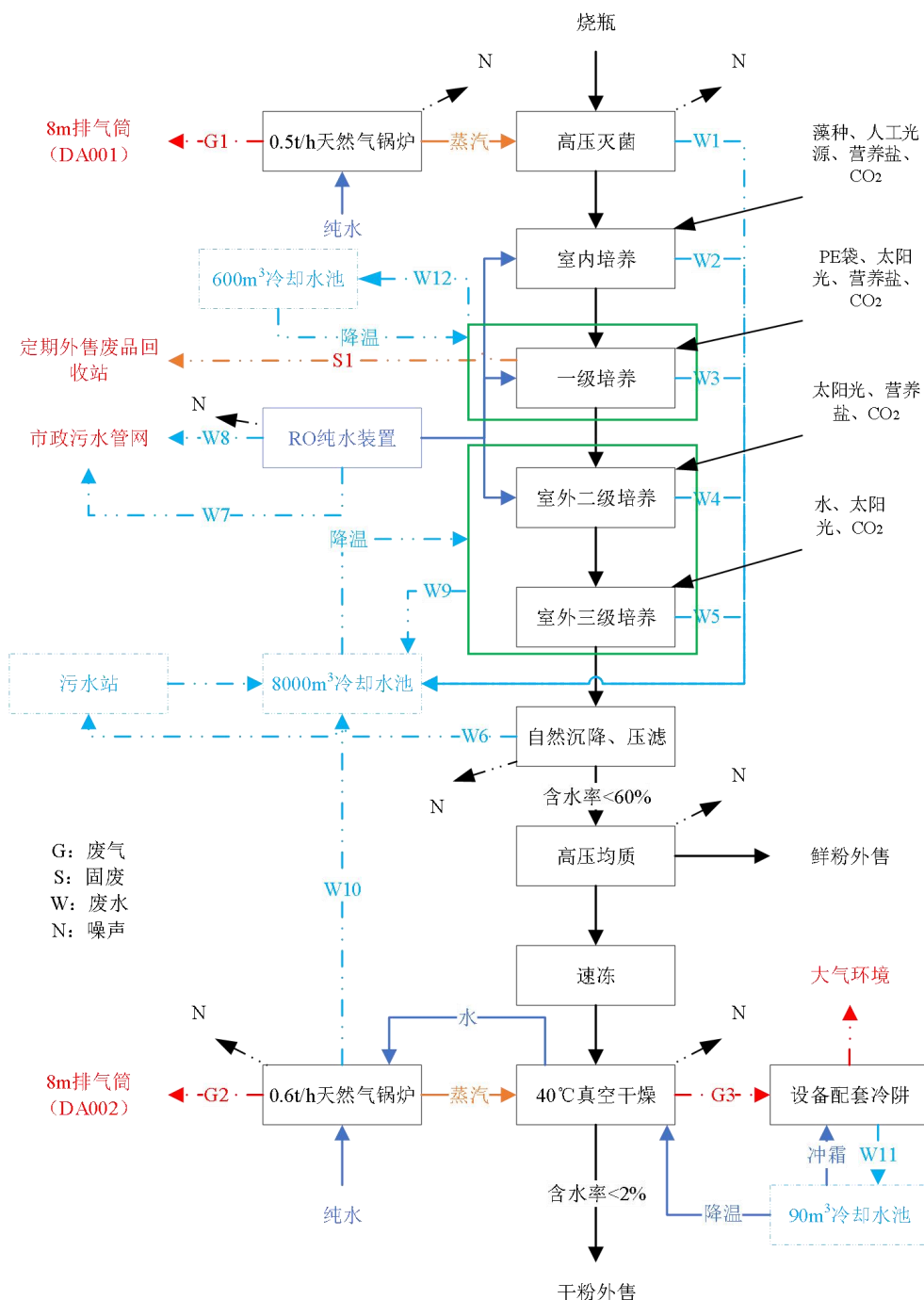
图 2-3 运营期工艺流程及产污环节图
