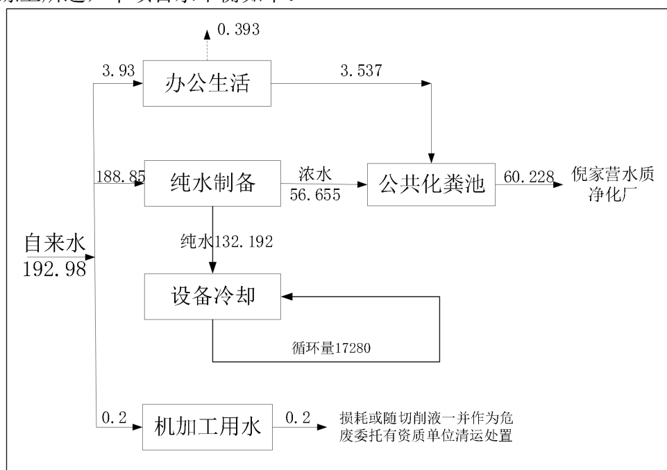
图 2-2 项目水量平衡图 单位：m 3 /d
