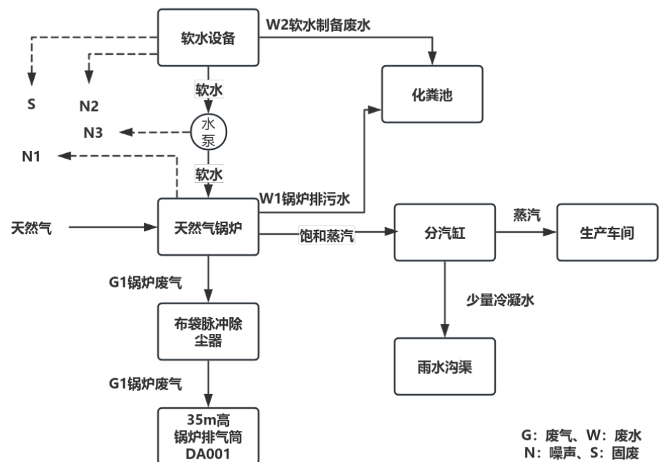
图 2-3 运营期锅炉生产工艺流程及产污环节示意图
