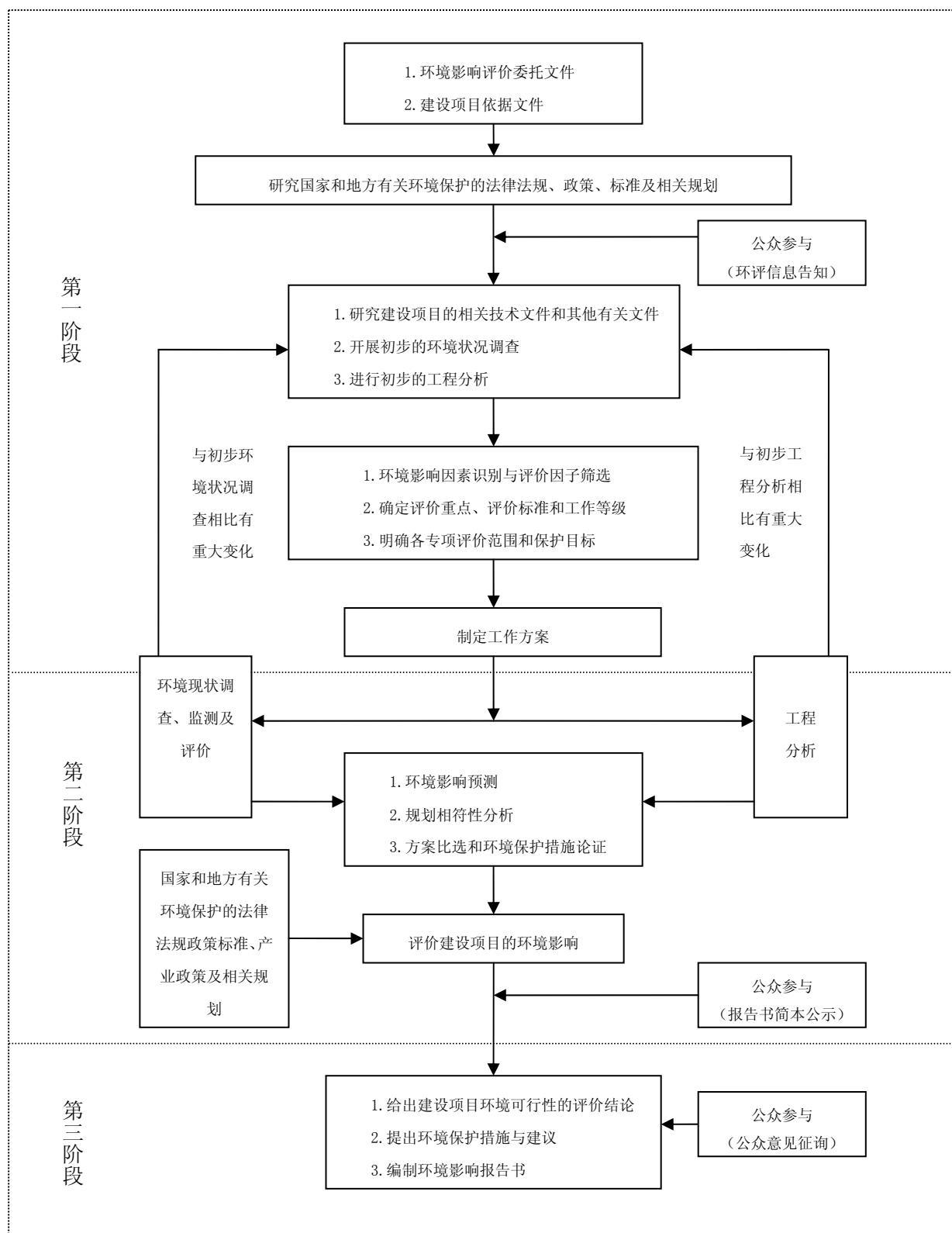
图 1 输变电工程环境影响评价的工作程序及内容
