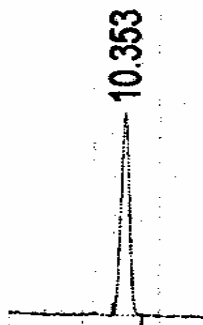
图 G.1 莠去津气相色谱图
